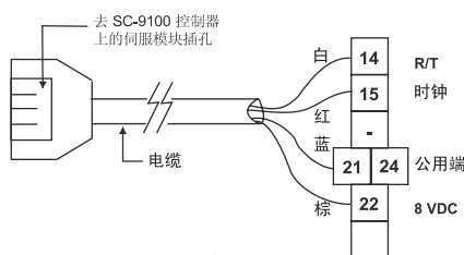
典型接线图
