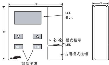
尺寸 (mm)
